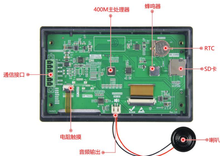
图 1-2 RS232 硬件配置图
