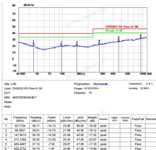
图 5-6 RE 测试水平方向
