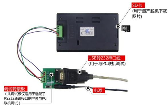
图 1-4 RS232 调试工具图
